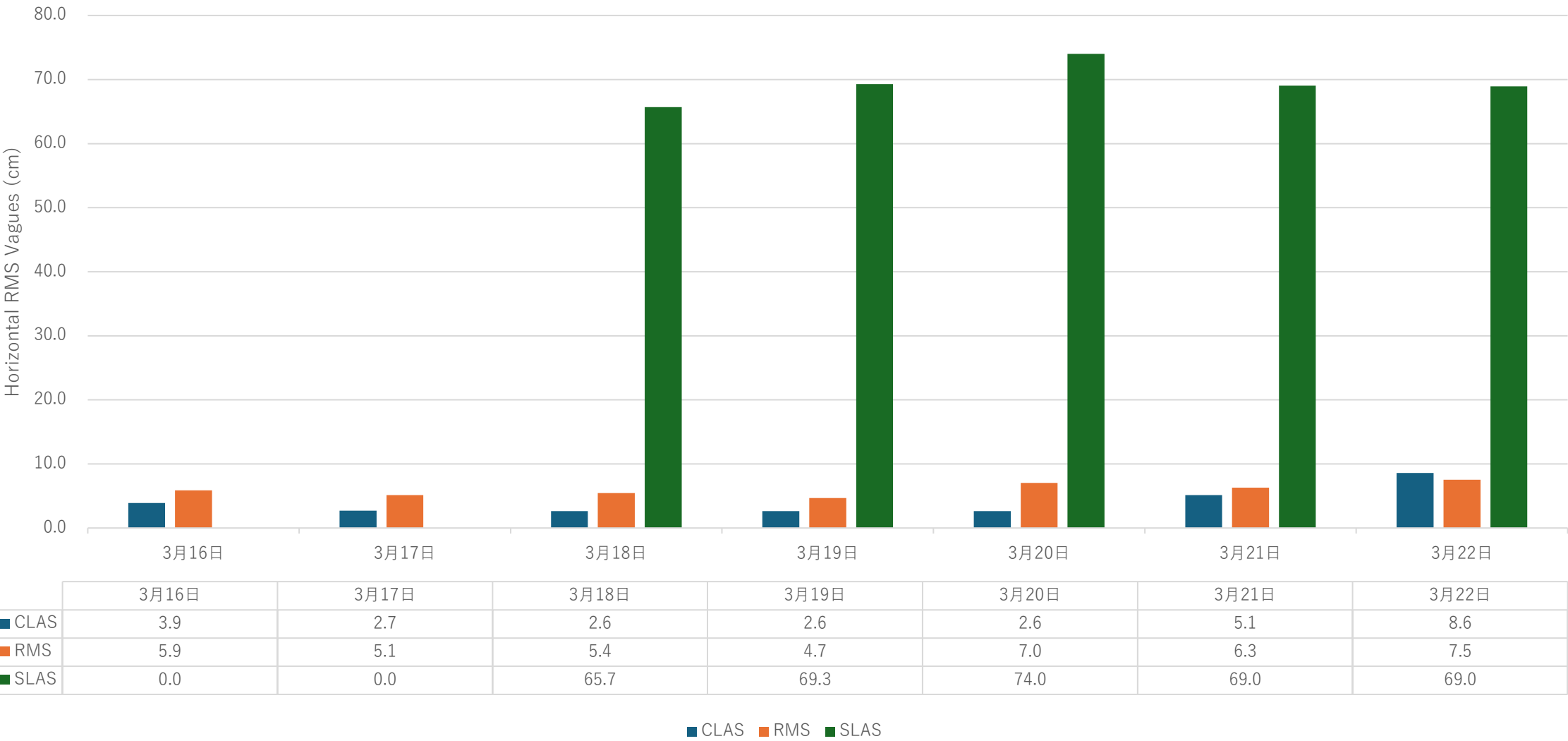
CLAS/PPP/SLASの水平RMS値 (2025/3/16– 2025/3/22)
