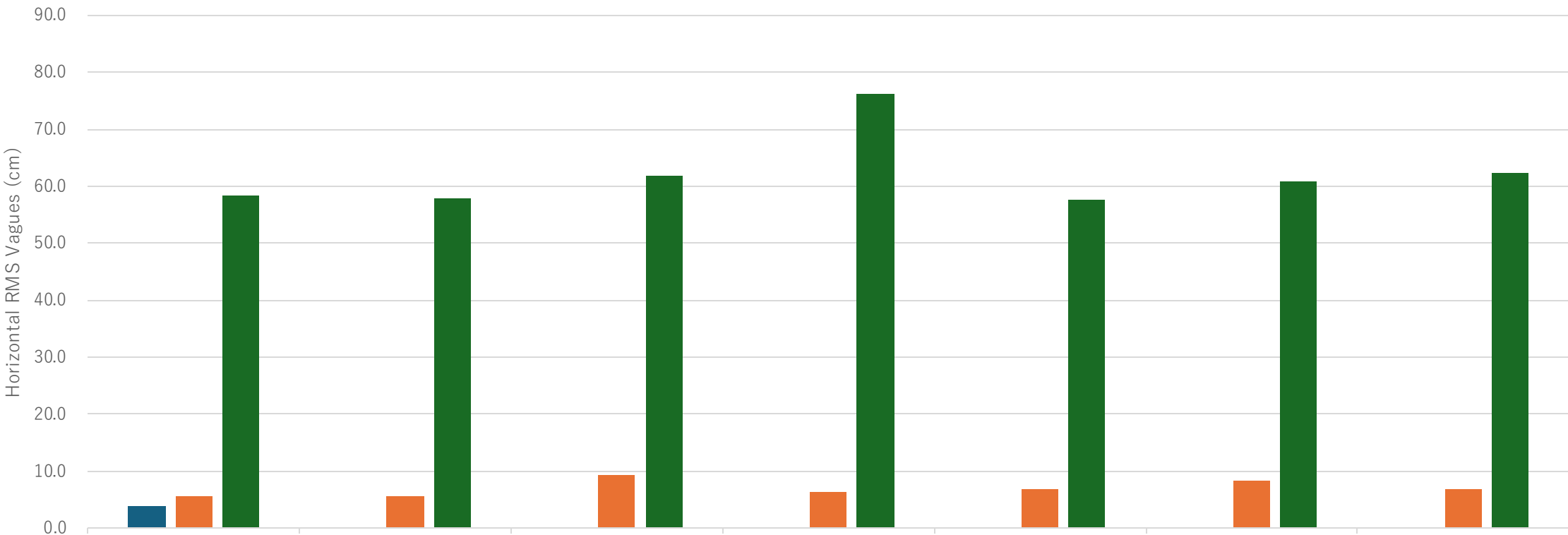
CLAS/PPP/SLASの水平RMS値 (2025/1/19– 2025/1/25)
