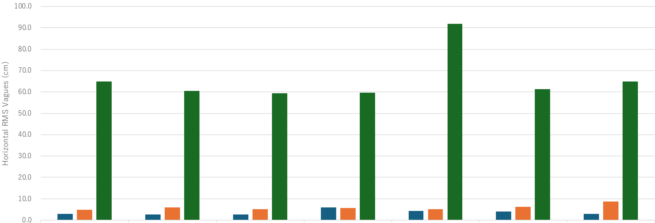
CLAS/PPP/SLASの水平RMS値 (2024/12/29– 2025/1/4)
