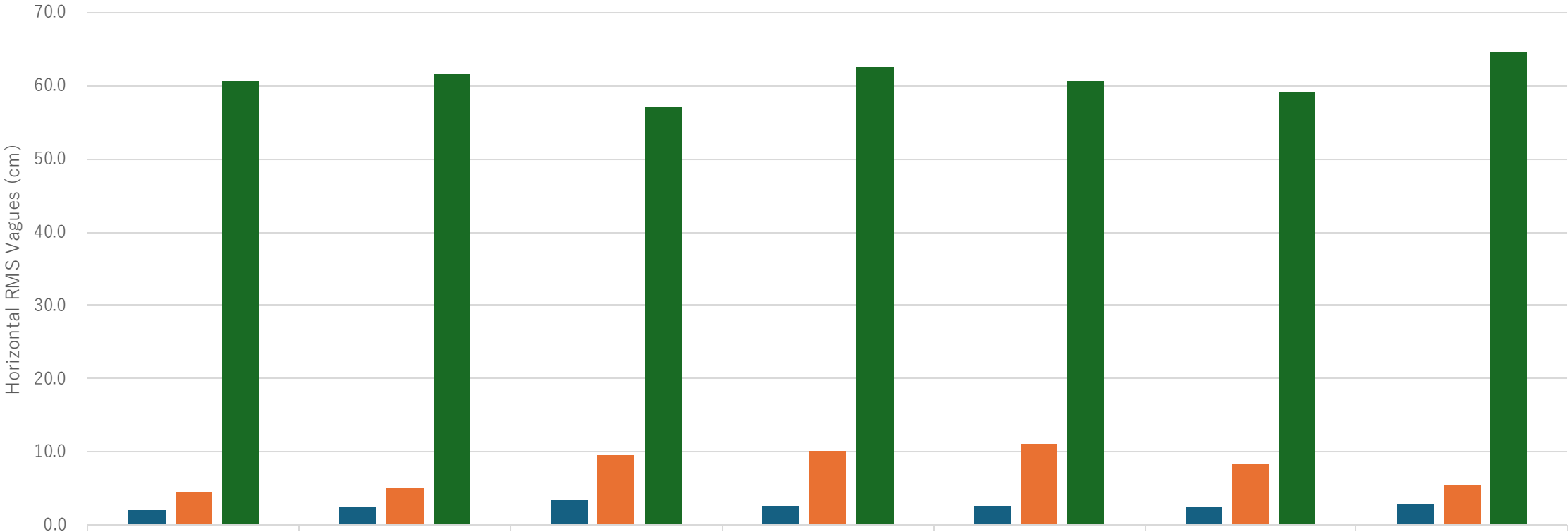
CLAS/PPP/SLASの水平RMS値 (2024/12/22- 2024/12/28)
