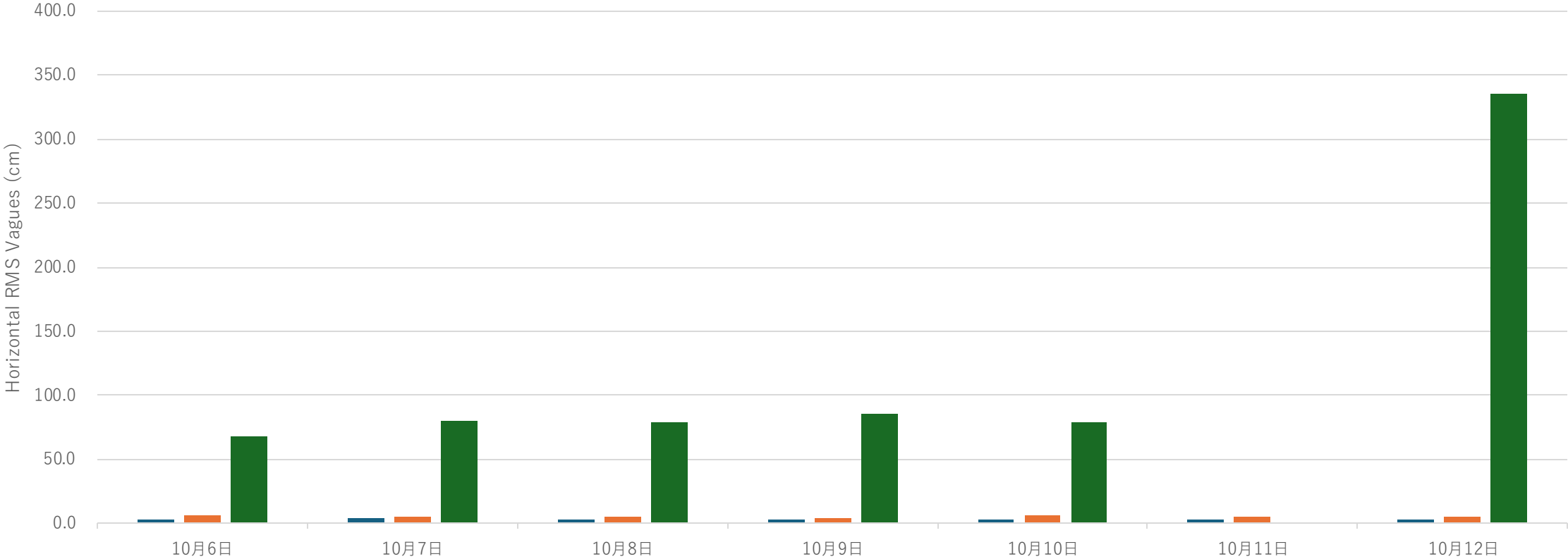
CLAS/PPP/SLASの水平RMS値 (2024/10/6– 2024/10/12)
