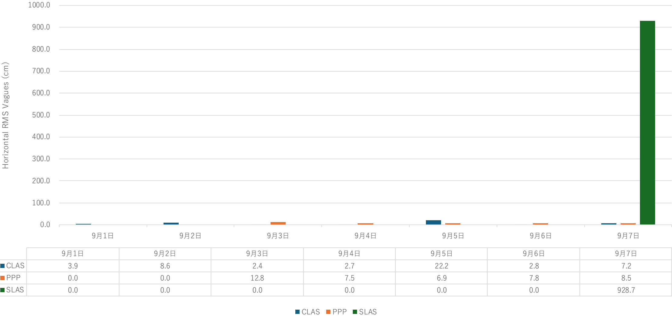
CLAS/PPP/SLASの水平RMS値 (2024/9/1– 2024/9/7)
