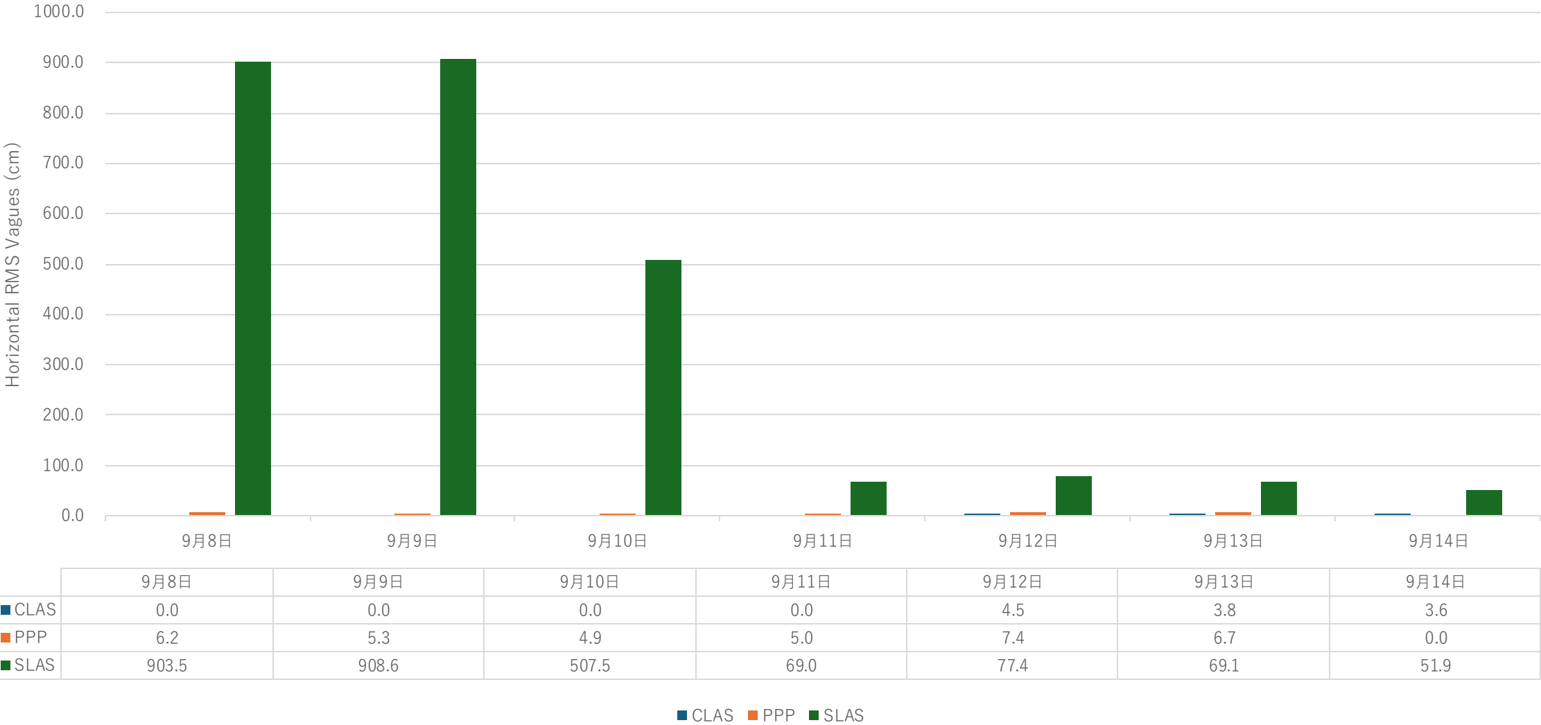
CLAS/PPP/SLASの水平RMS値 (2024/9/8– 2024/9/14)
