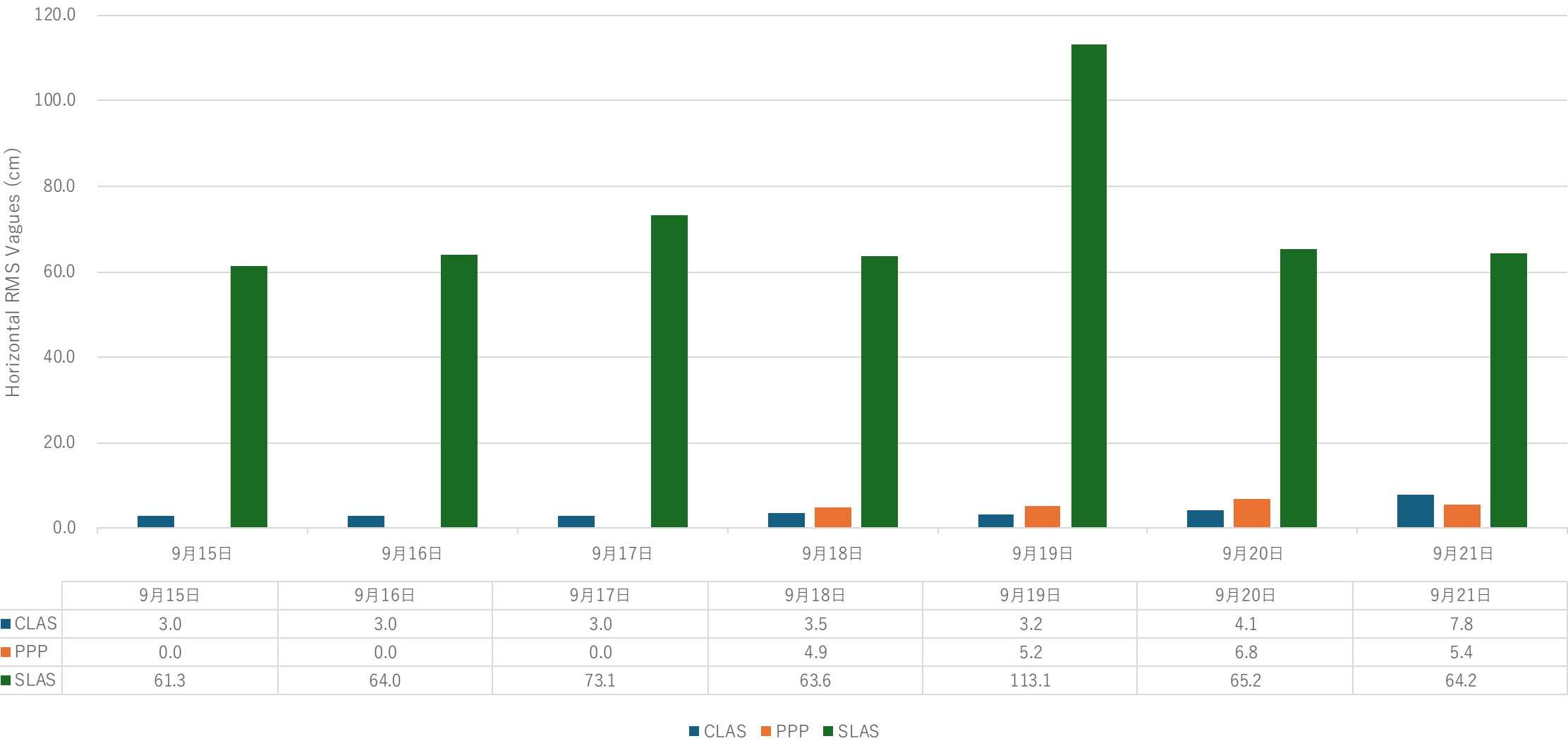
CLAS/PPP/SLASの水平RMS値 (2024/9/15– 2024/9/21)
