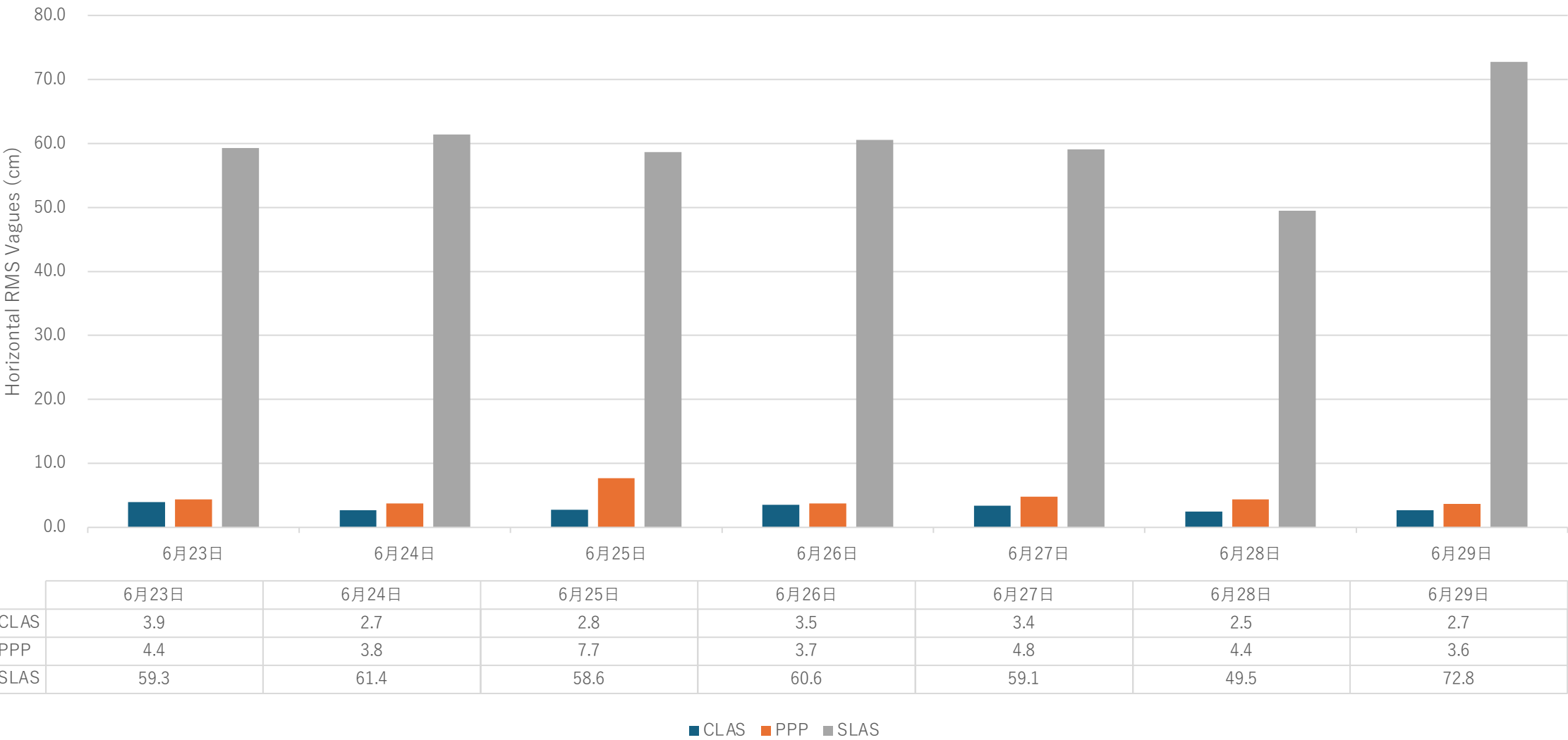
CLAS/PPP/SLASの水平RMS値 (2024/6/23– 2024/6/29)
