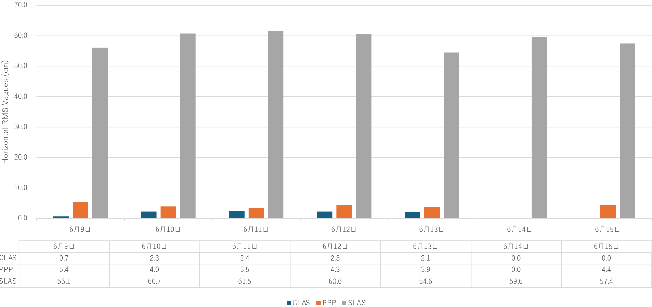
CLAS/PPP/SLASの水平RMS値 (2024/6/9– 2024/6/15)
