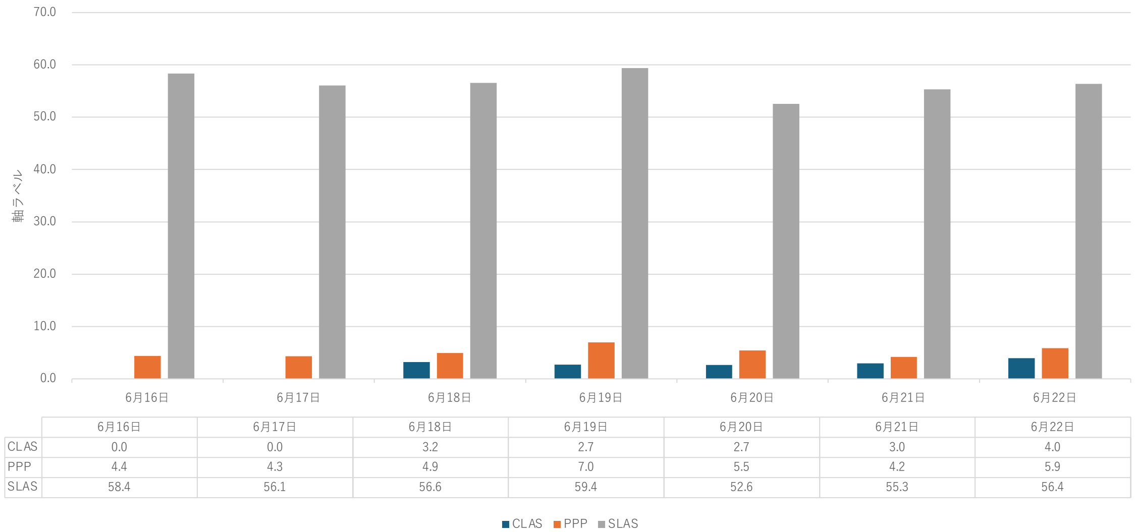
CLAS/PPP/SLASの水平RMS値 (2024/6/16– 2024/6/22)
