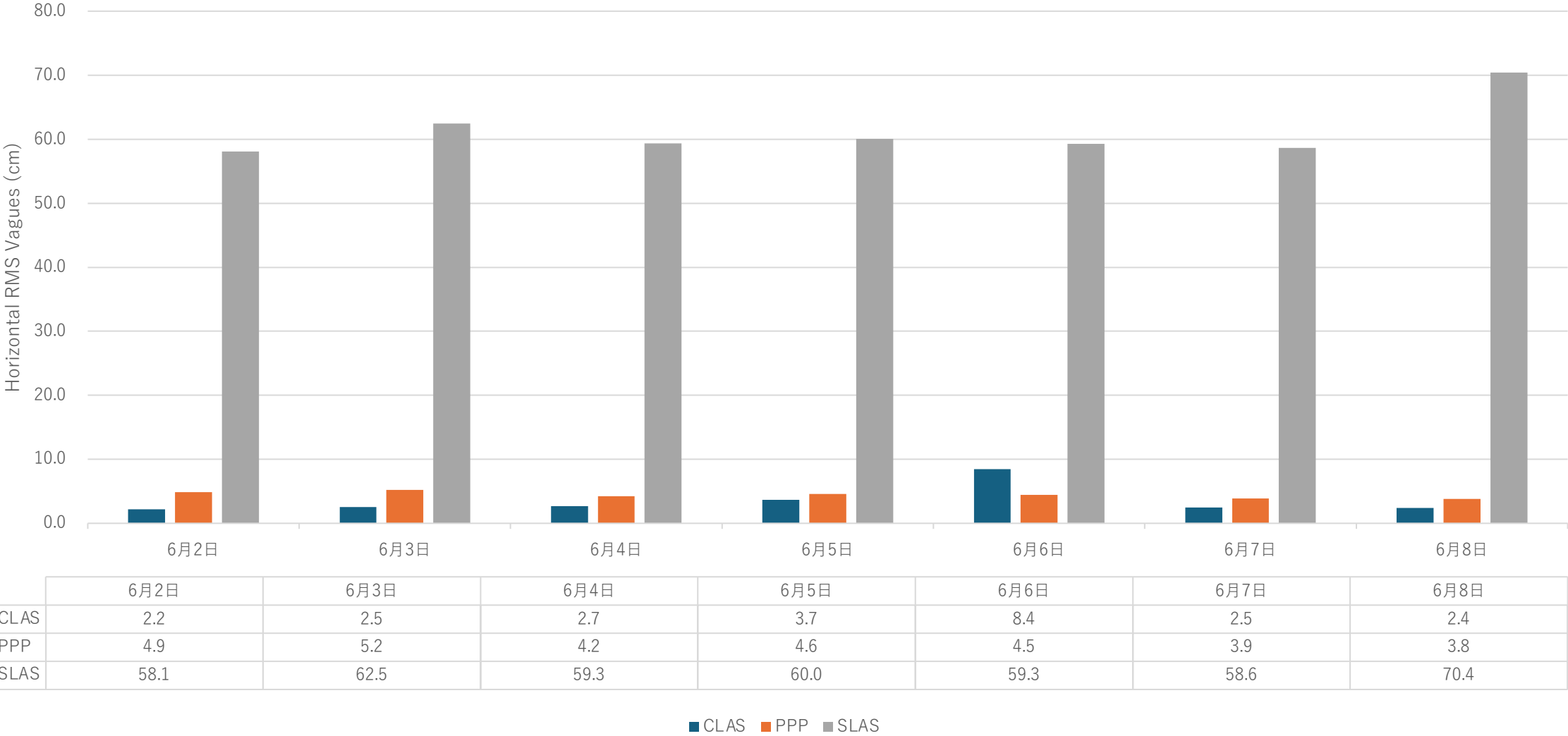
CLAS/PPP/SLASの水平RMS値 (2024/6/2- 2024/6/8)
