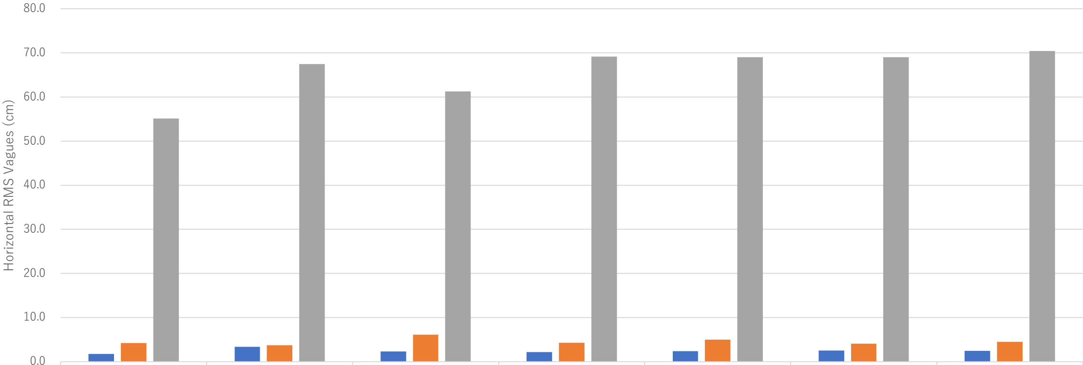
CLAS/PPP/SLASの水平RMS値 (2024/4/21– 2024/4/27)
