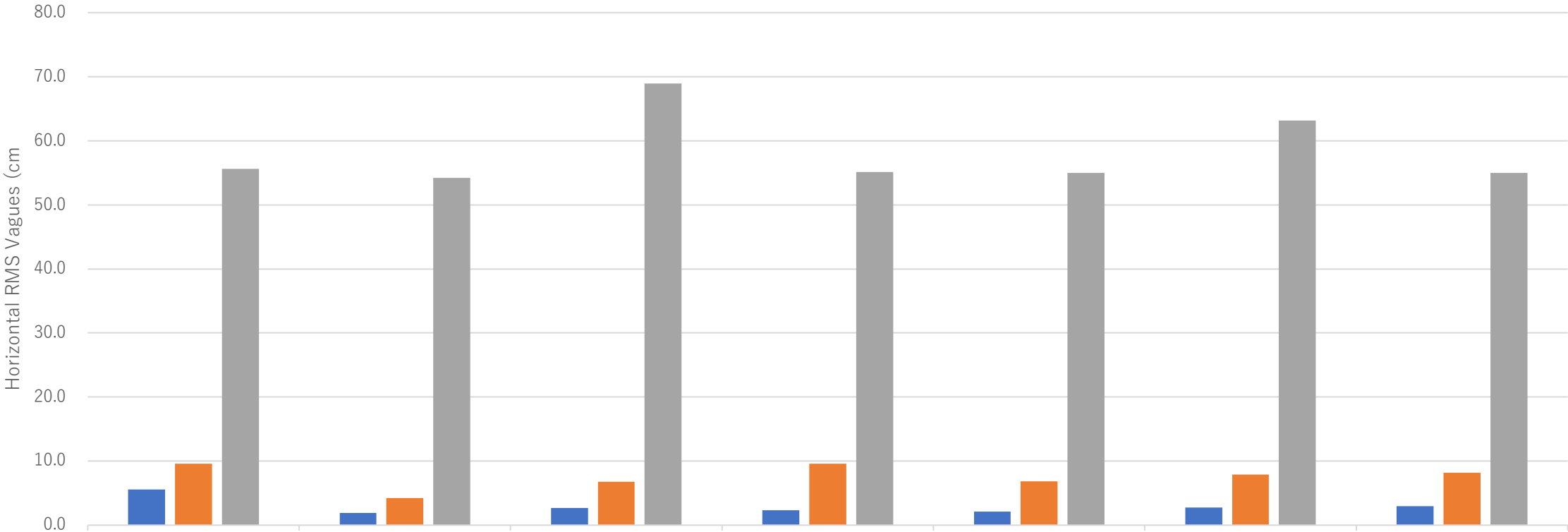
CLAS/PPP/SLASの水平RMS値 (2024/2/4– 2024/2/10)
