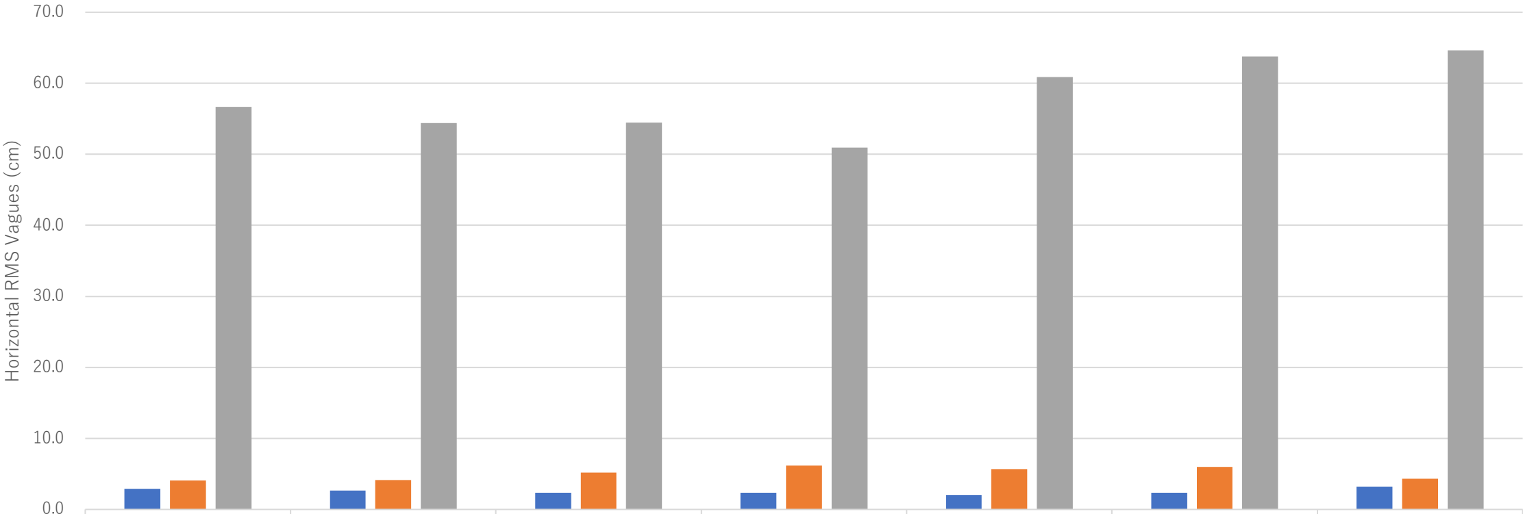
CLAS/PPP/SLASの水平RMS値 (2024/2/18– 2024/2/24)
