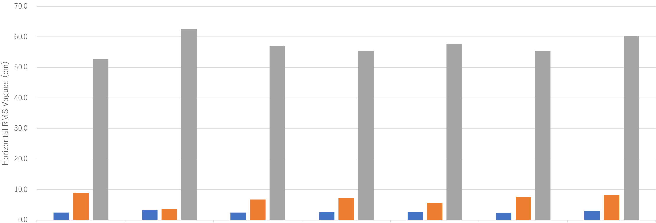
CLAS/PPP/SLASの水平RMS値 (2024/2/11– 2024/2/17)
