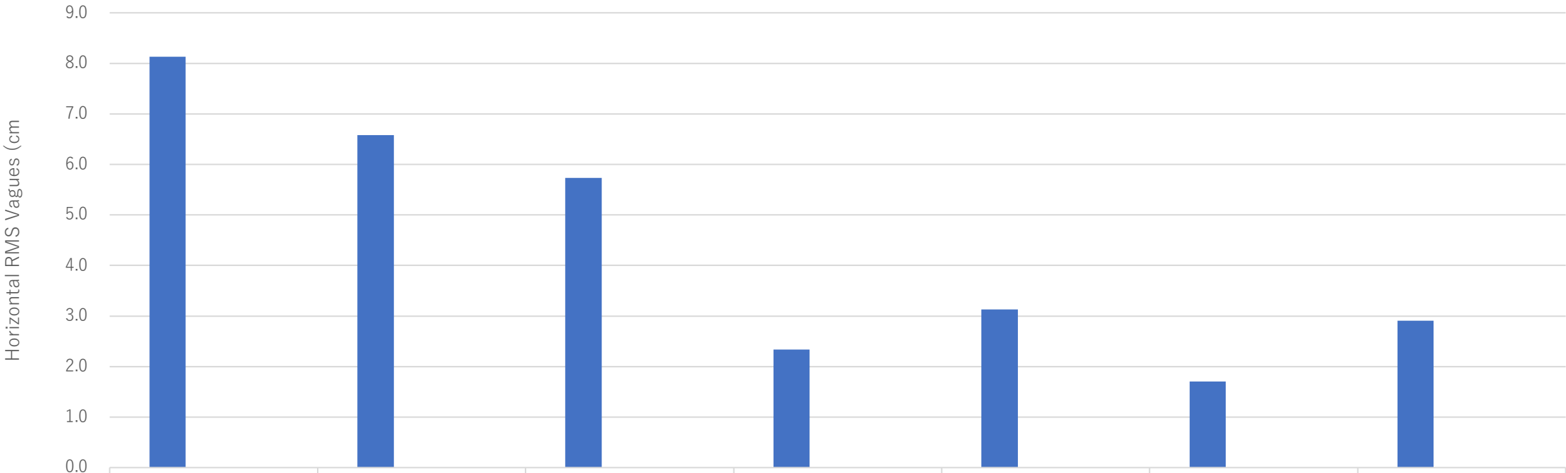
CLAS/PPP/SLASの水平RMS値 (2023/12/3– 2023/12/9)
